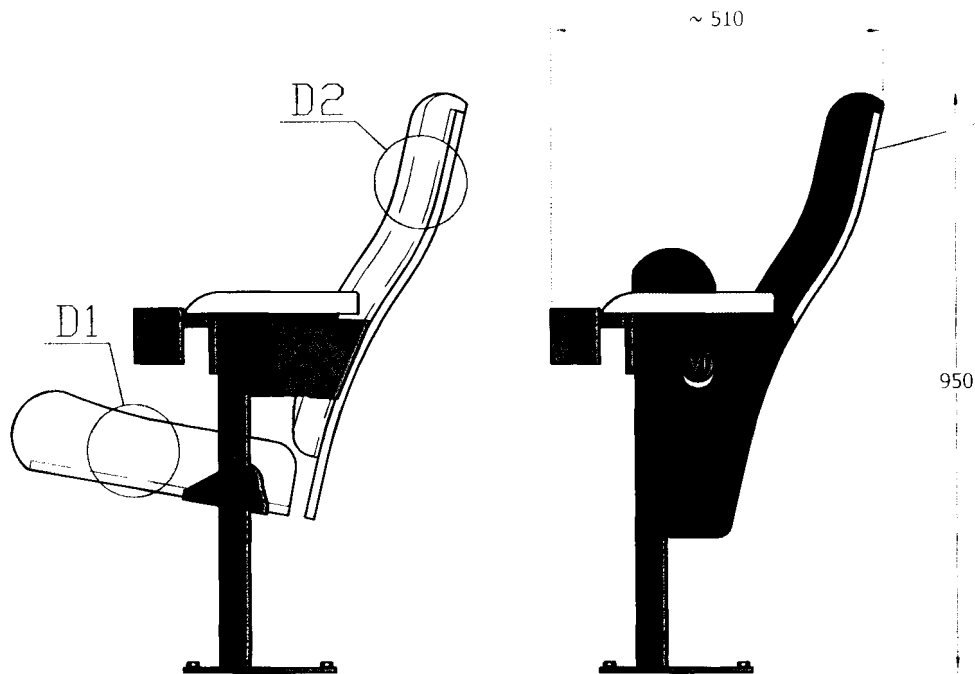
DET.D1-SEDÁK
