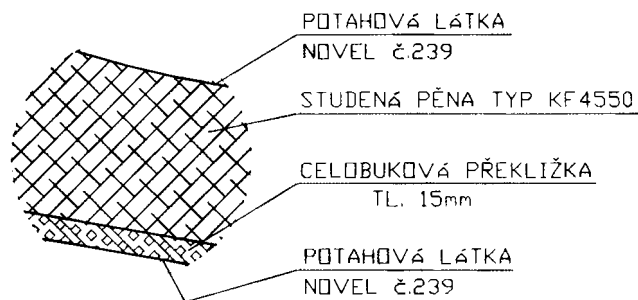
DET.D1-SEDÁK
